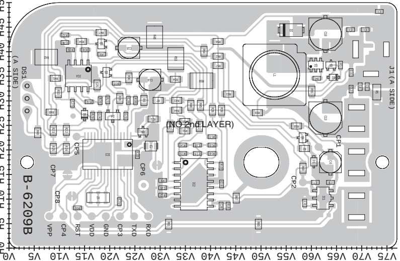
• BC-160 (TOP VIEW)
